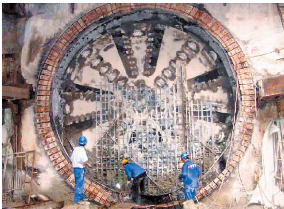
盾构区间贯通时盾构机顺利冲出的瞬间。时报通讯员 常青 彭明汉 沈靖宇 摄
