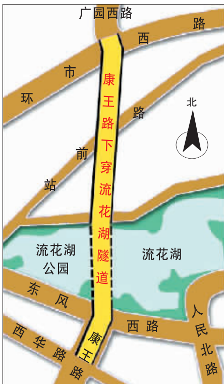
隧道示意图
